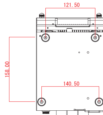
【底面】
