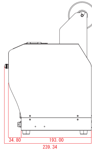
【右面】
