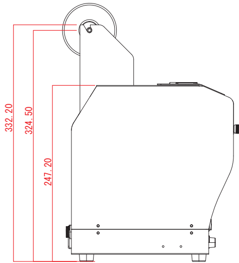
【左面】
